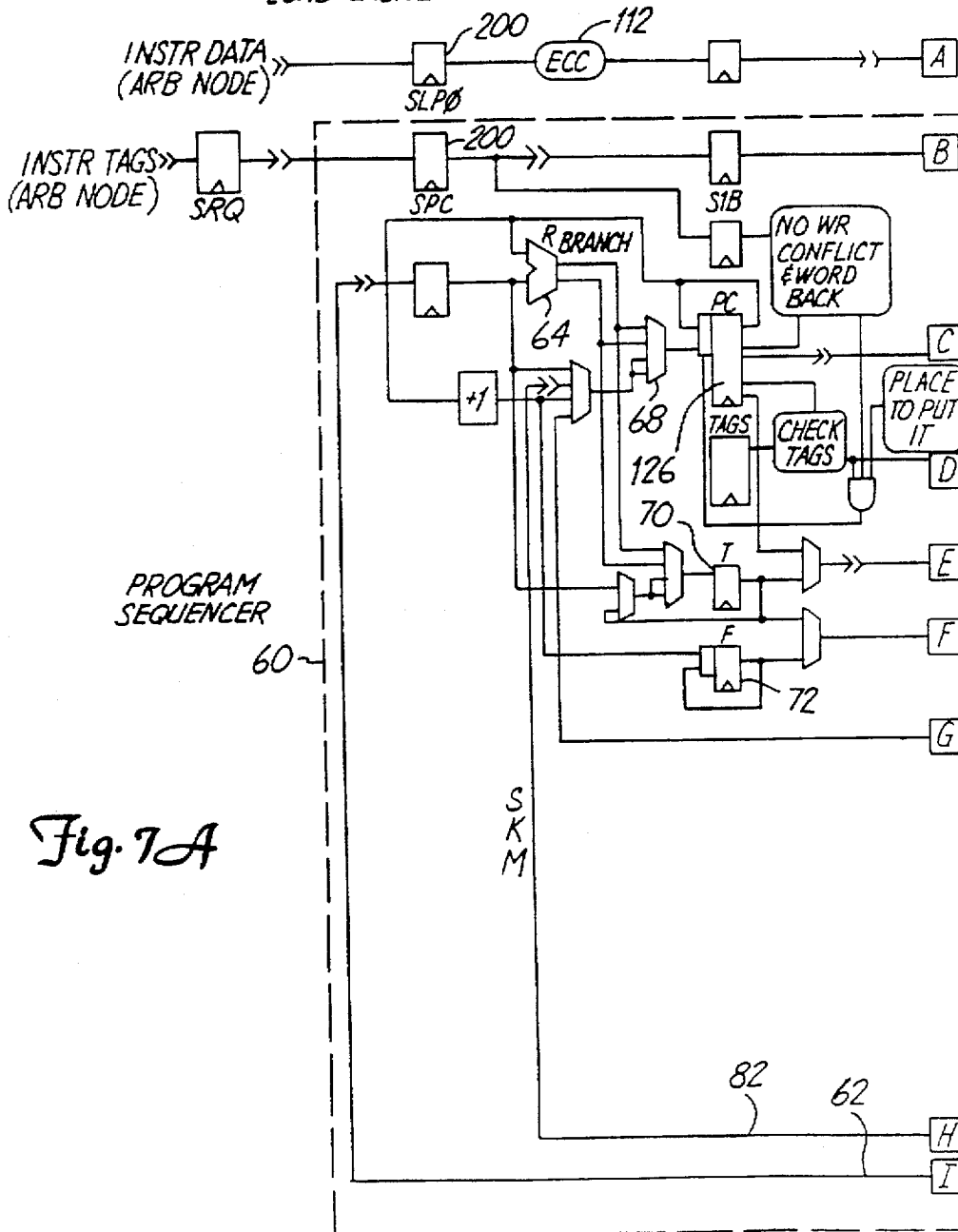
INSTR LOAD CACHE Fig. 7
