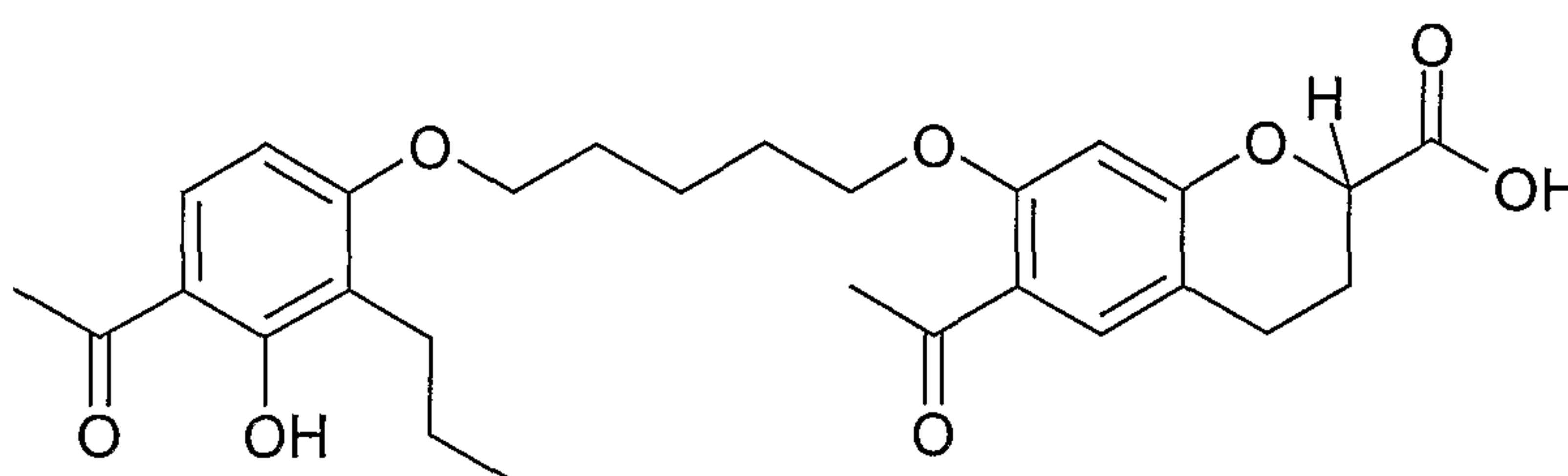
Ablukast
