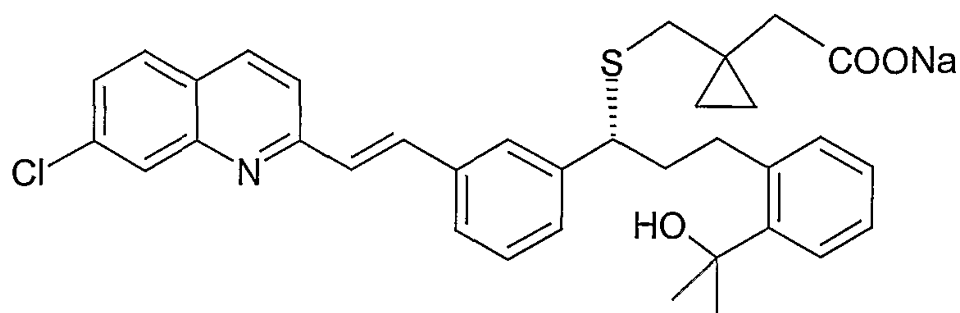
Montekulast
