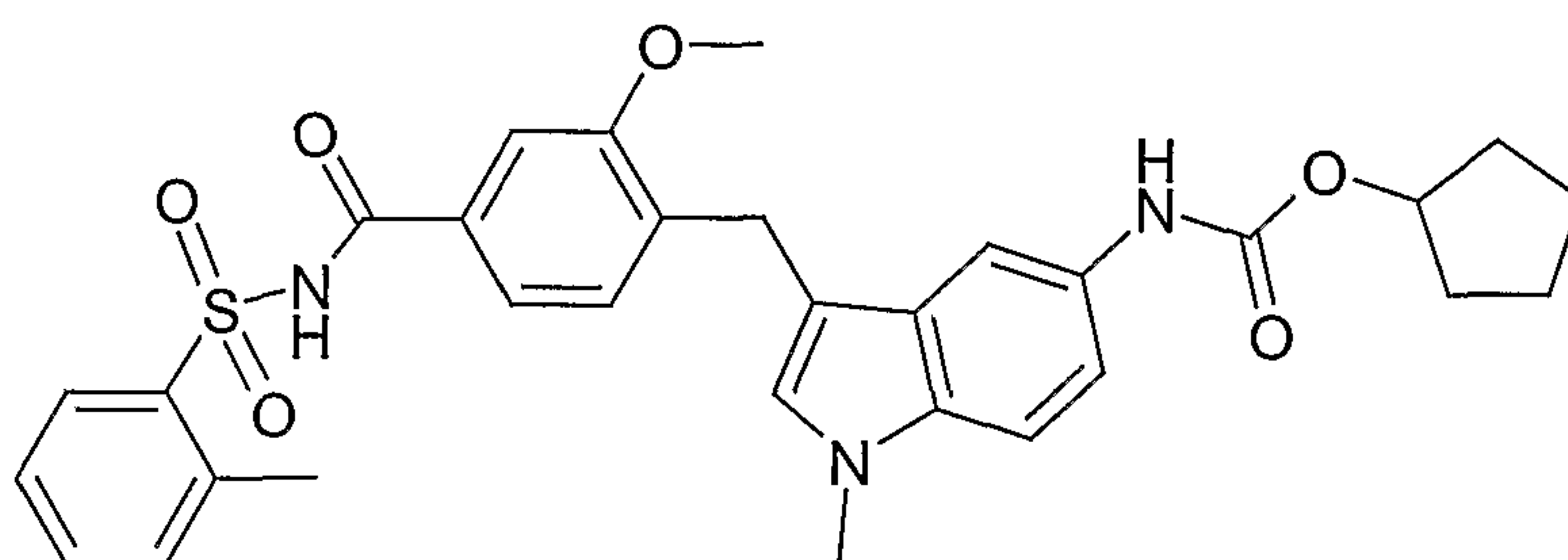
Zafirlukast
