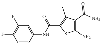
5-Amino-N2-(3,4-difluorophenyl)-3-methylthiophene-2,4-dicarboxamide (ZW-896)
