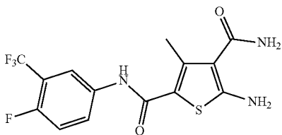
5-Amino-N2-(4-fluoro-3-(trifluoromethyl)phenyl)-3-methylthiophene-2,4-dicarboxamide (ZW-1057)
