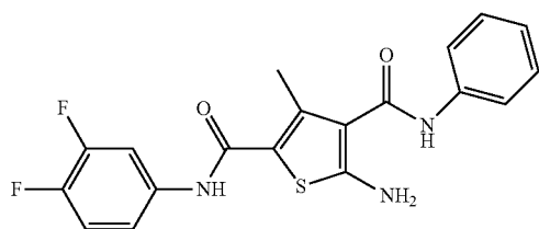
5-Amino-N2-(3,4-difluorophenyl)-3-methyl-N4-phenylthiophene-2,4-dicarboxamide (ZW-892)
