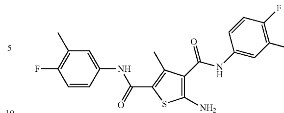
5-Amino-N2,N4-bis(4-fluoro-3-methylphenyl)-3-methylthiophene-2,4-dicarboxamide (ZW-1070)
