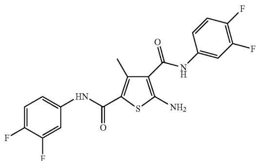
5-Amino-N2,N4-bis(3,4-difluorophenyl)-3-methylthiophene-2,4-dicarboxamide (ZW-932)
