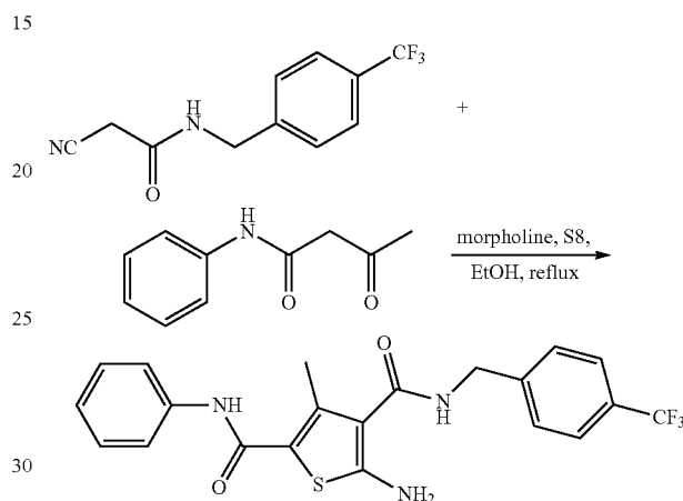
5-Amino-3-methyl-N2-phenyl-N4-(4-(trifluoromethyl)benzyl)thiophene-2,4-dicarboxamide (ZW-790)
