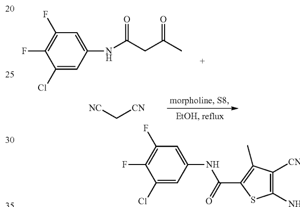
5-Amino-N-(3-chloro-4,5-difluorophenyl)-4-cyano-3-methylthiophene-2-carboxamide (ZW-1042)
