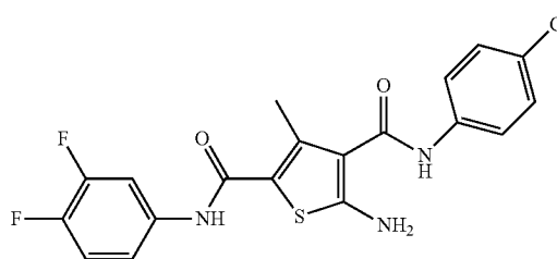
5-Amino-N4-(4-chlorophenyl)-N2-(3,4-difluorophenyl)-3-methylthiophene-2,4-dicarboxamide (ZW-893)
