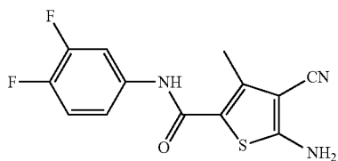
5-Amino-4-cyano-N-(3,4-difluorophenyl)-3-methylthiophene-2-carboxamide (ZW-1043)
