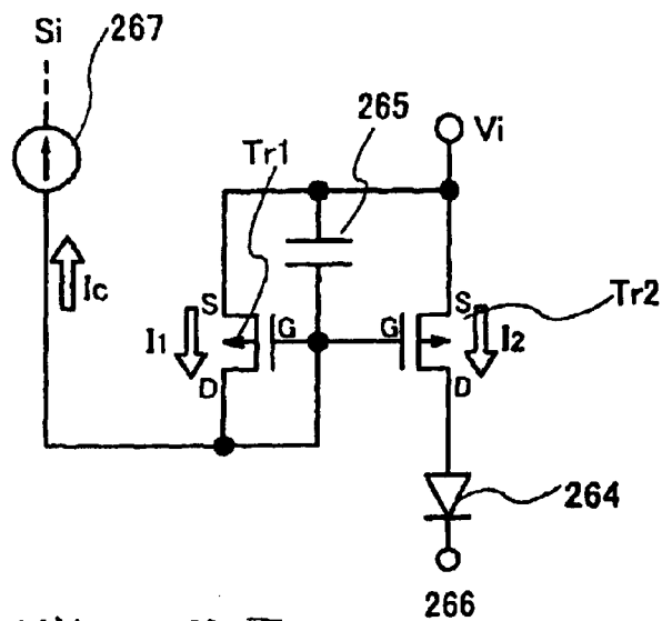
FIG. 25B DISPLAY PERIOD T_d
