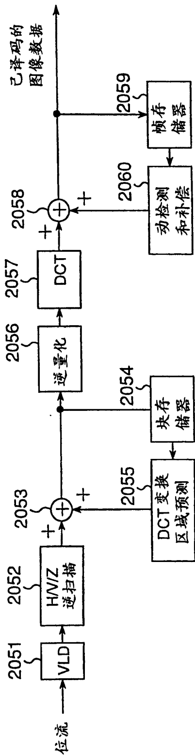
实施例8 图像预测译码装置
