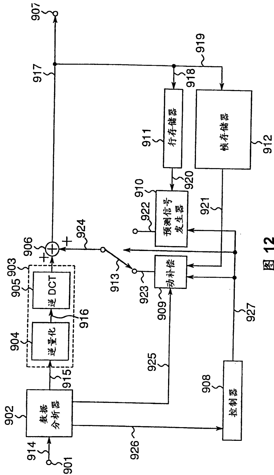
实施例3 图像预测译码装置
