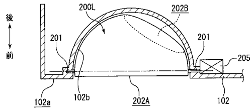
(A) 第1状態 (A-A断面図)
