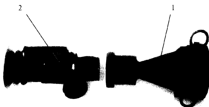
Fig. 12. Modul de cuplare a Adaptorului 4x pe Monocularul de vedere/ ochire pe timp de noapte – WOLF 1x
