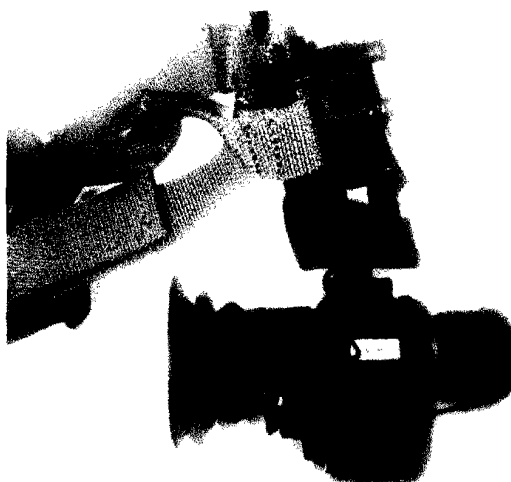
Fig. 10. Monocular de vedere/ ochire pe timp de noapte – WOLF 1x fixat pe Dispozitivul de prindere pe casca NATO
