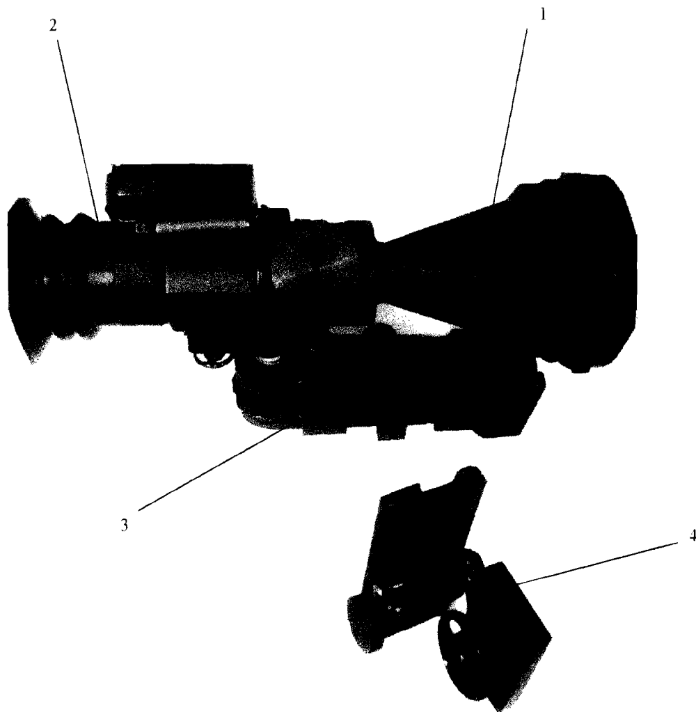
Fig. 1. Sistem multifunctional de observare si ochire pe timp de noapte - WOLF
