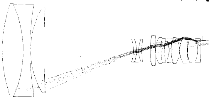
Fig. 3 Adaptor 4x cuplat cu obiectivul monocularului - Schema optică
