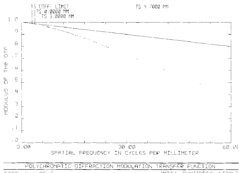
Fig. 5 Funcția optică de transfer pentru: - Adaptor 4x cuplat cu obiectivul monocularului - distanța obiect 15 m
