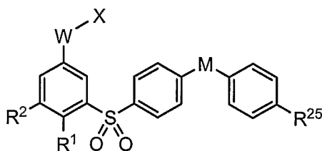
Formula Im
