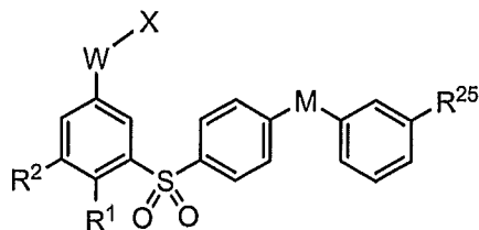
Formula Ik
