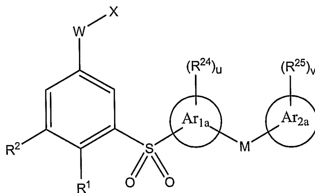
Formula Ic
