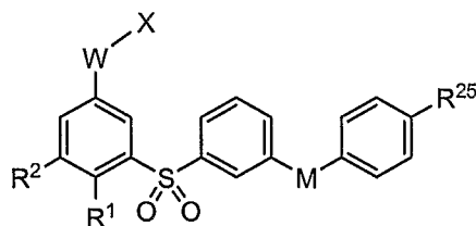
Formula Ij
