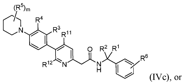
(IVa),
