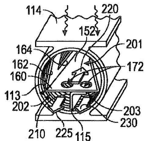
FIG. 6A (Section A-A)
