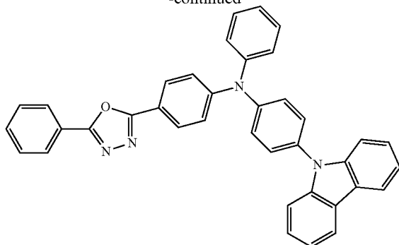
YGAO11
