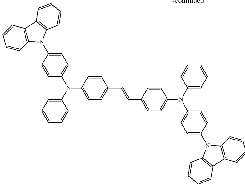
YGA2S
