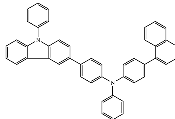
PCBANB
