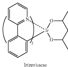
Ir(ppy) 2 acac
