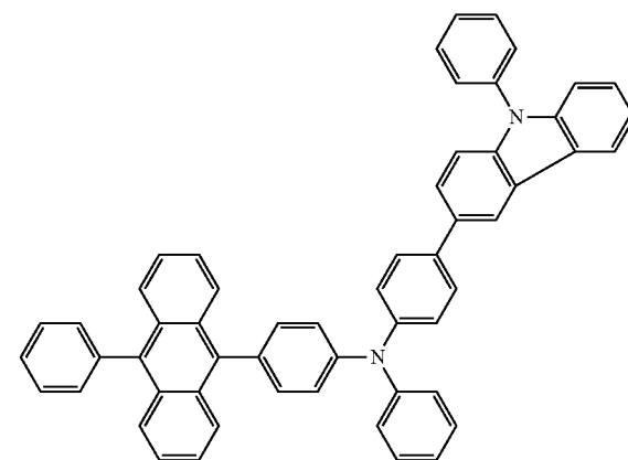
PCBAPA
