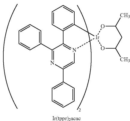
Ir(tppr) 2 acac
