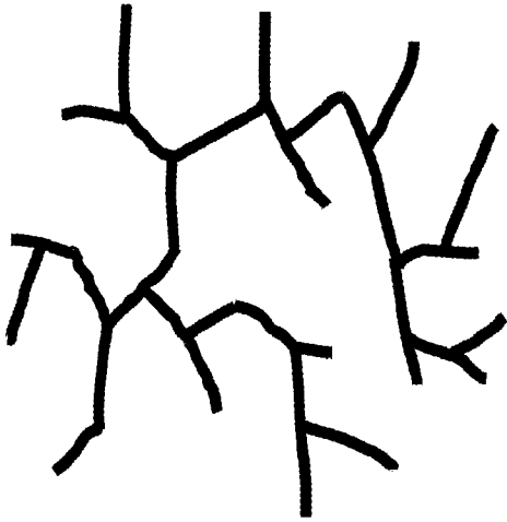
Random ABP
