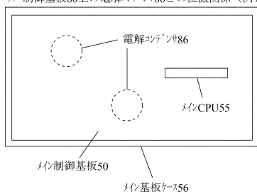
(b) メイン制御基板50上のメインCPU55とサブ制御基板80上の電解コンデンサ86との位置関係 (例2)
