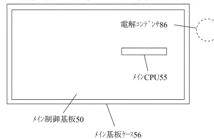
(d) メイン制御基板50上のメインCPU55とサブ制御基板80上の電解コンデンサ86との位置関係 (例4)
