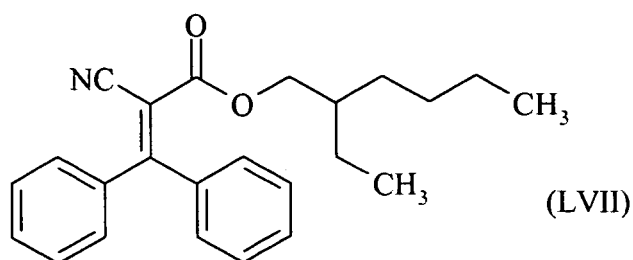
(2-Ethylhexyl)-2-cyano-3,3-diphenylacrylate
