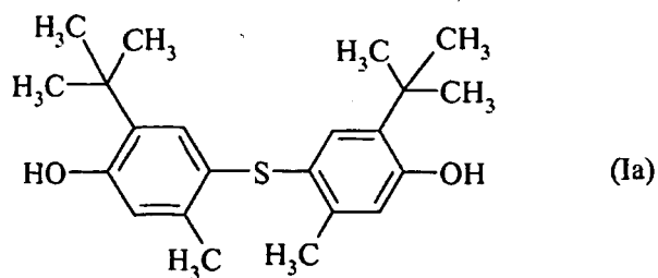
4,4'-thiobis-(6-tert.-butyl-m-crésol)
