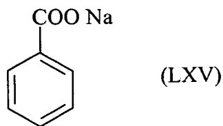
Sodiumbenzoate
