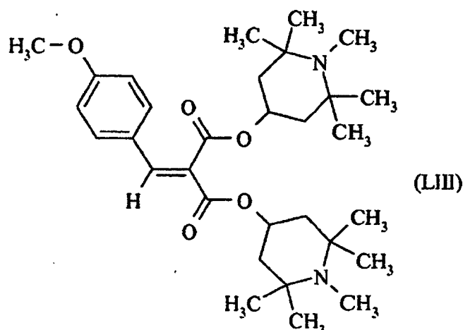
Propandisäure[(4-methoxyphenyl)methylen]bis(1,2,2,6,6-pentamethyl-4-piperidinyl)ester
