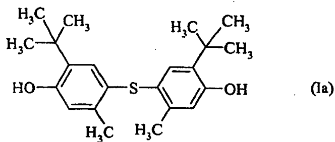
4,4'-Thiobis(6-tert.-butyl-m-kresol)
