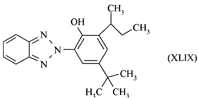
2-(2H-benzotriazol-2-yl)-4-(tert-butyl)-6-(sec-butyl)phenol
