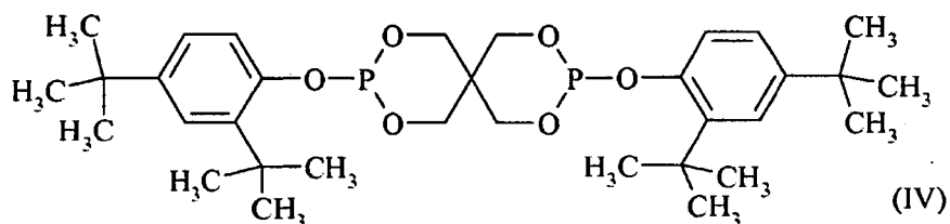
bis(2,4-di-t-butylphényl)pentaérythritol diphosphite
