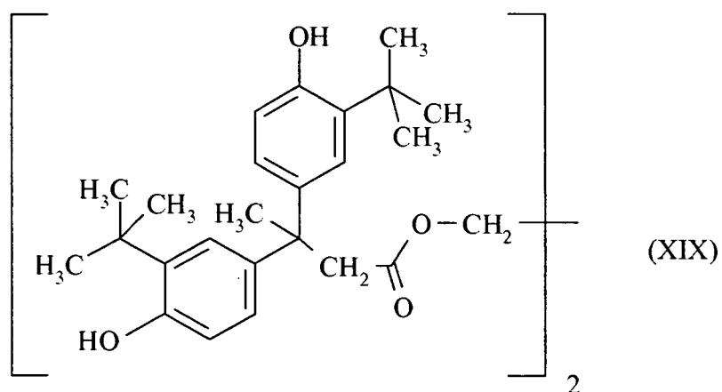
Bis[3,3-bis-(4'-hydroxy-3'-tert-butylphenyl)butanoicacid]-glycolester
