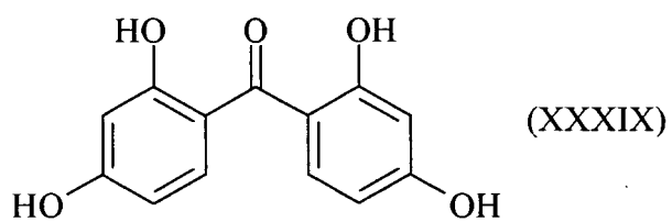
2,2',4,4'-Tetrahydroxybenzophenone
