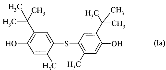
4,4'-thiobis-(6-tert.-butyl-m-cresol)
