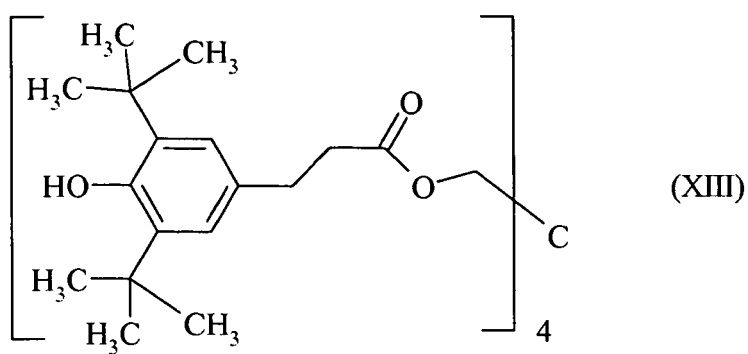
Tetrakis[methylene(3,5-di-tert-butylhydroxyhydrocinnamate)]-methane
