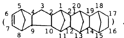
Nonacyclo[1 11,11 ,1 5,8 ,1 13,20 ,1 15,18 ,0 2,10 ,0 4,9 0 12,21 ,0 14,19 ]-eicos-6-ene
