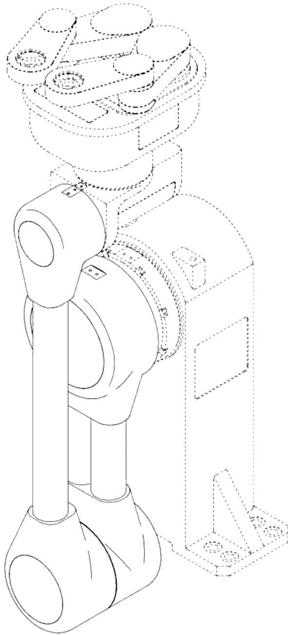
【立體圖】
