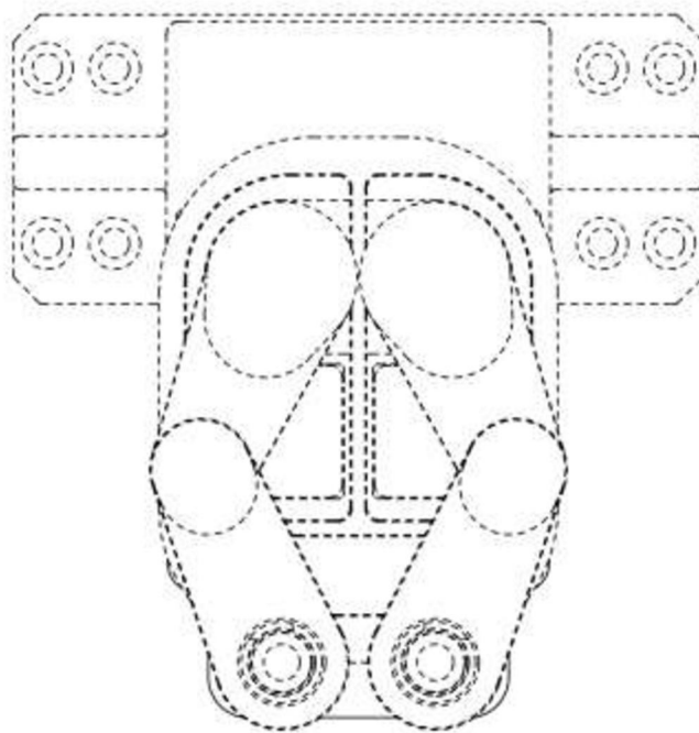
【俯視圖】
