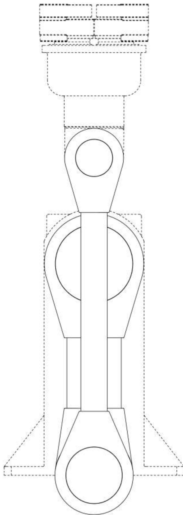
【前視圖】
