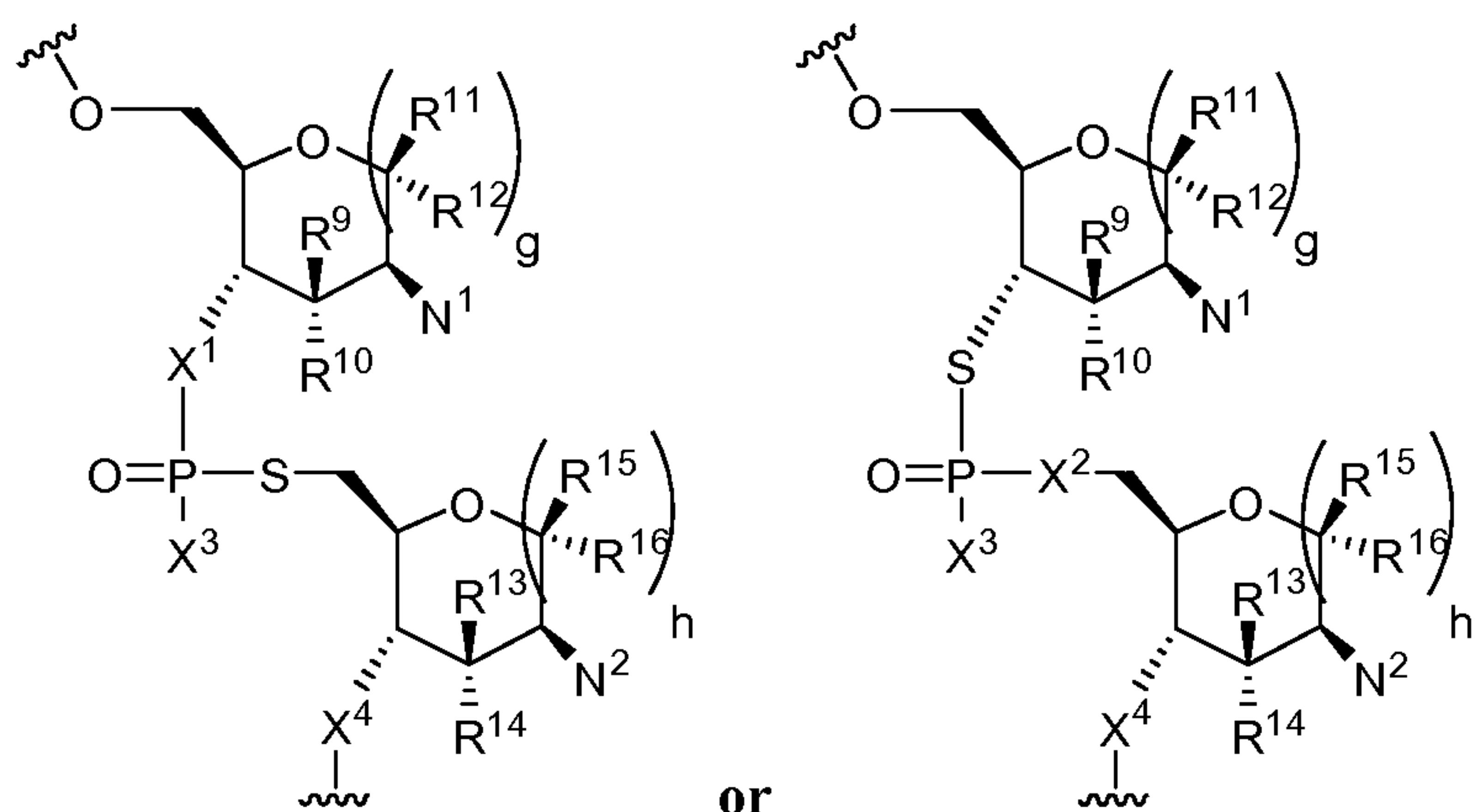
Formula Va
