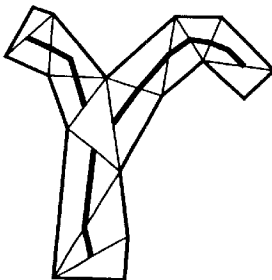
(d) Construction of Chordal Axis
