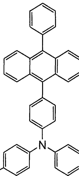
PCBAPA (11)
