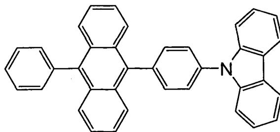
CzPA
