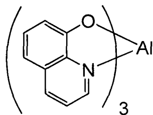
Alq 3
