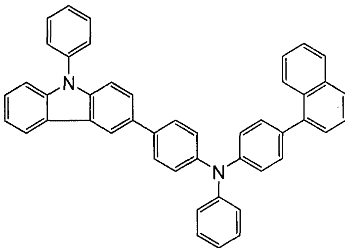
PCBANB (12)
