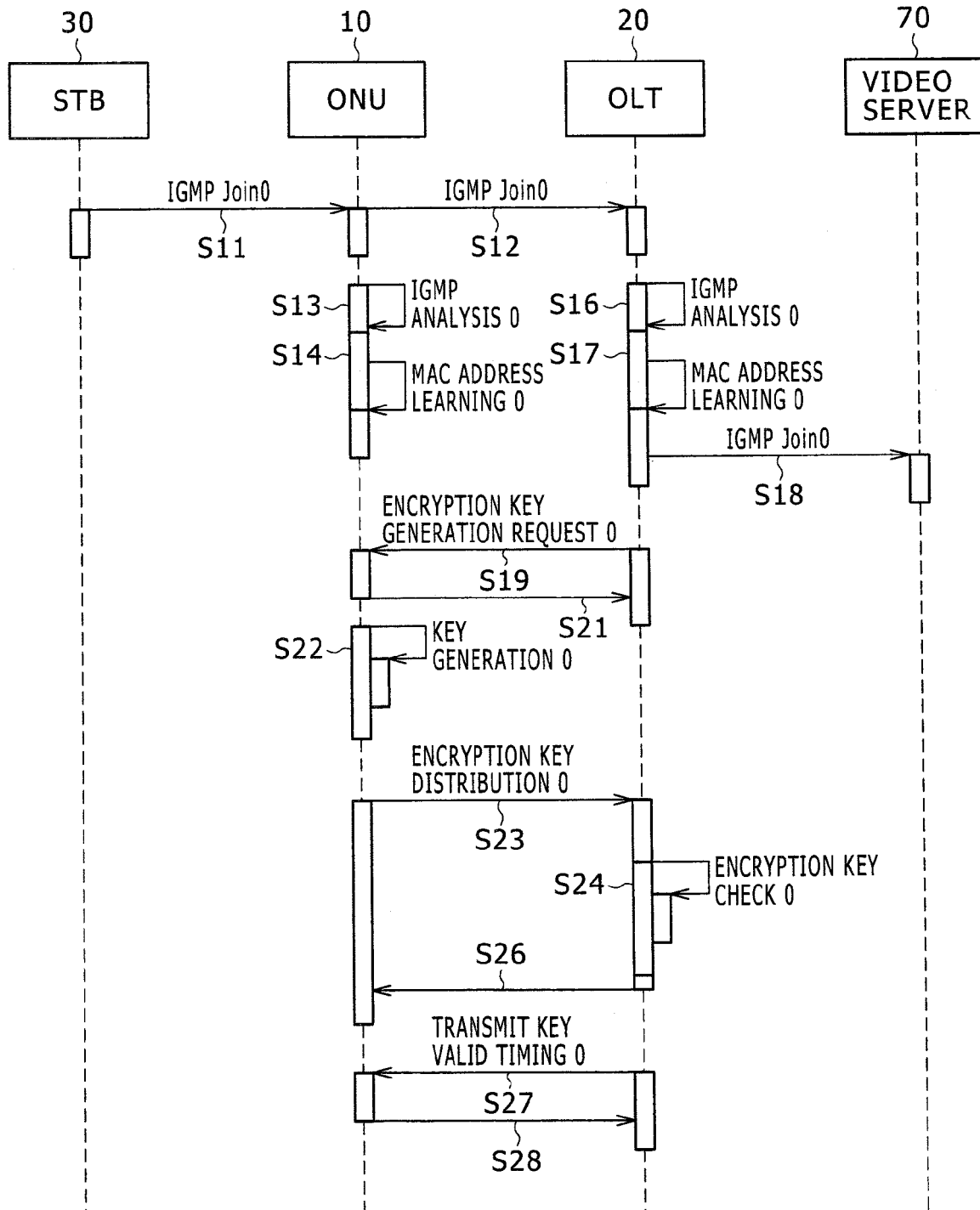
FIG. 8A
