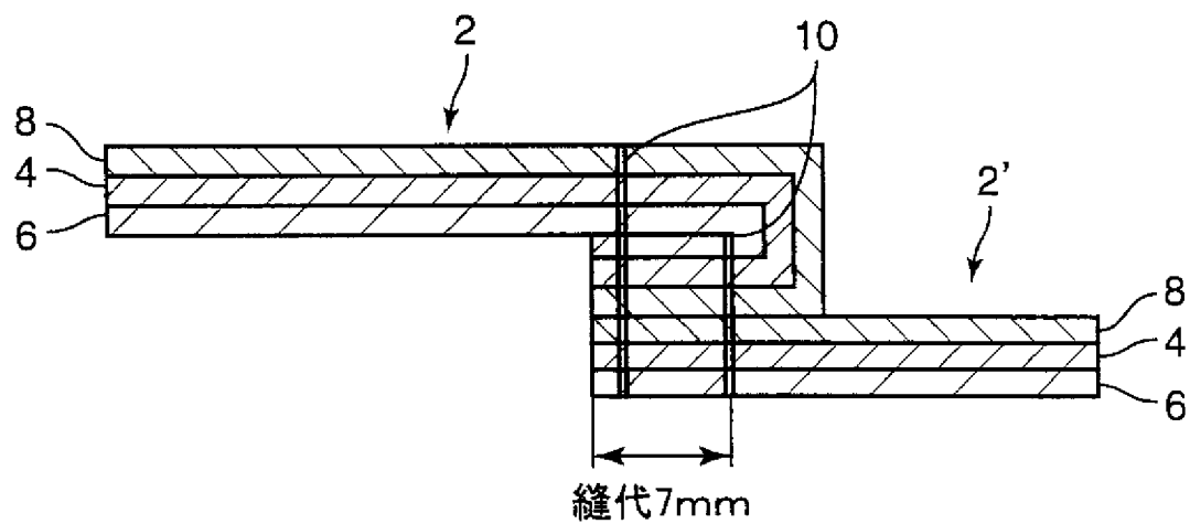
接合部断面図(X-X' 断面)
