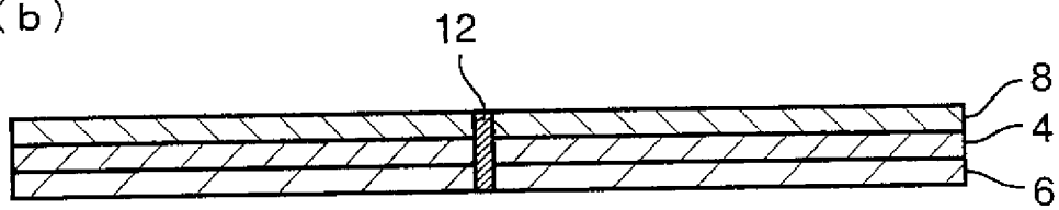
接合部断面図(X-X' 断面)
