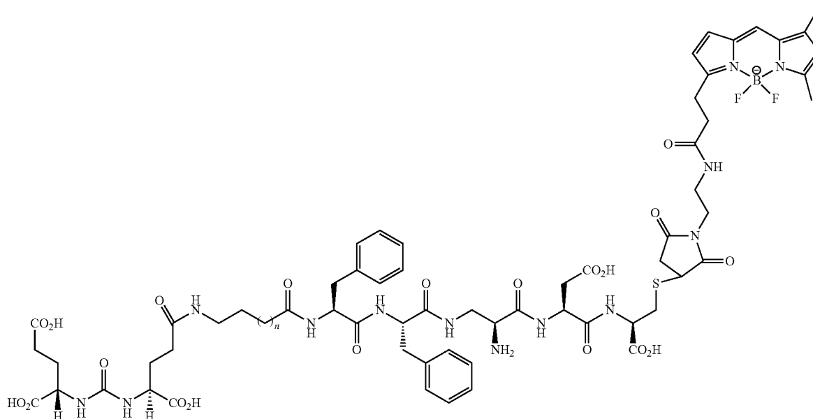
SK45 (25 Atom Linker BODIPY 505, C 67 H 87 BF 2 N 13 O 20 S, Mol. Wt.: 1475.35)
