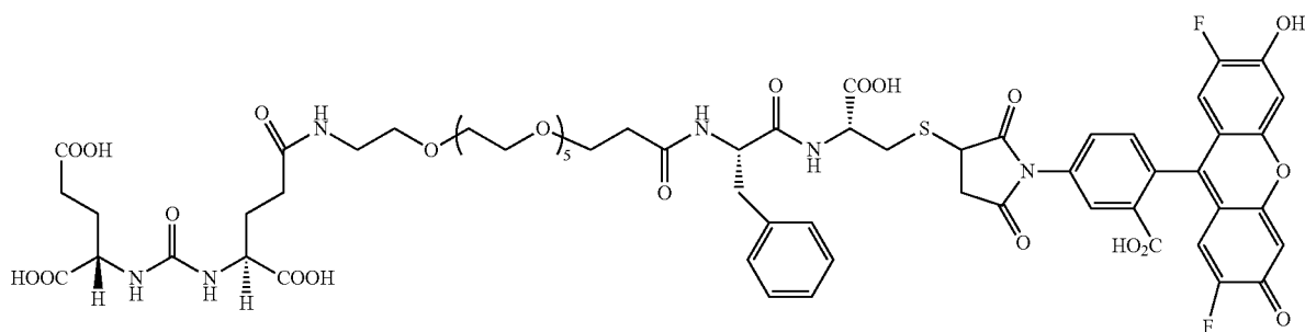
PC01SK56 C_{62}H_{70}F_2N_6O_{25}S Mol. Wt.: 1369.31
