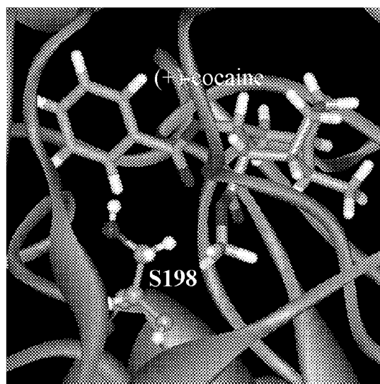
(D) BChE-(+)-cocaine prereactive complex
