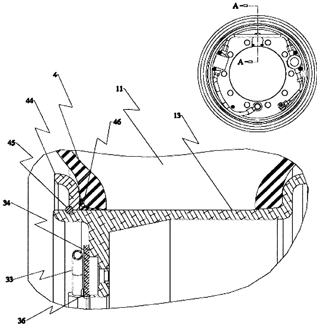
FIG. 11 (SECTION A-A)
