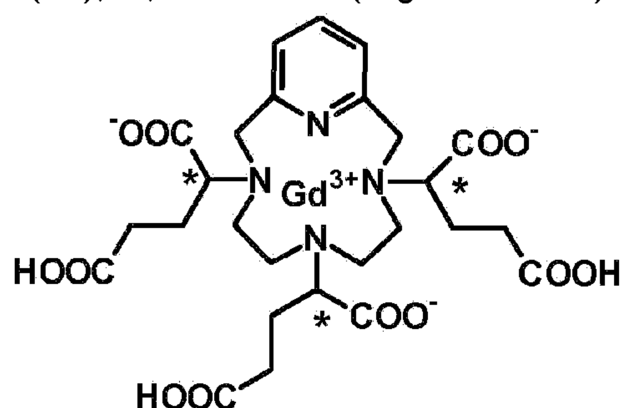
Gd(PCTA-tris-glutaric acid)
