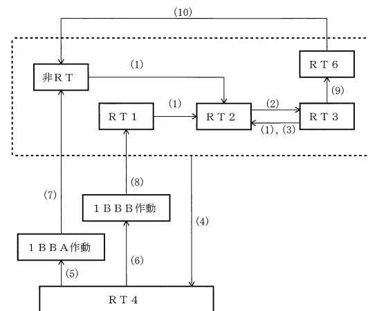
&lt;第6実施形態:RT移行図&gt;
