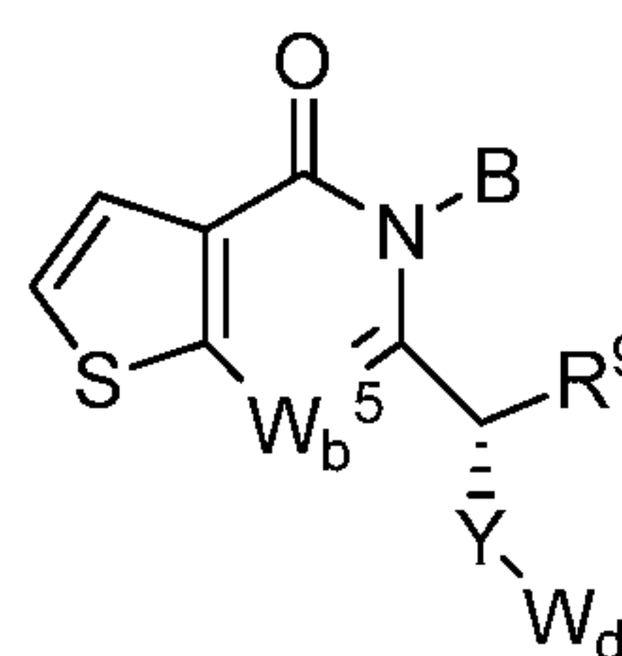
Formula (VIIb).
