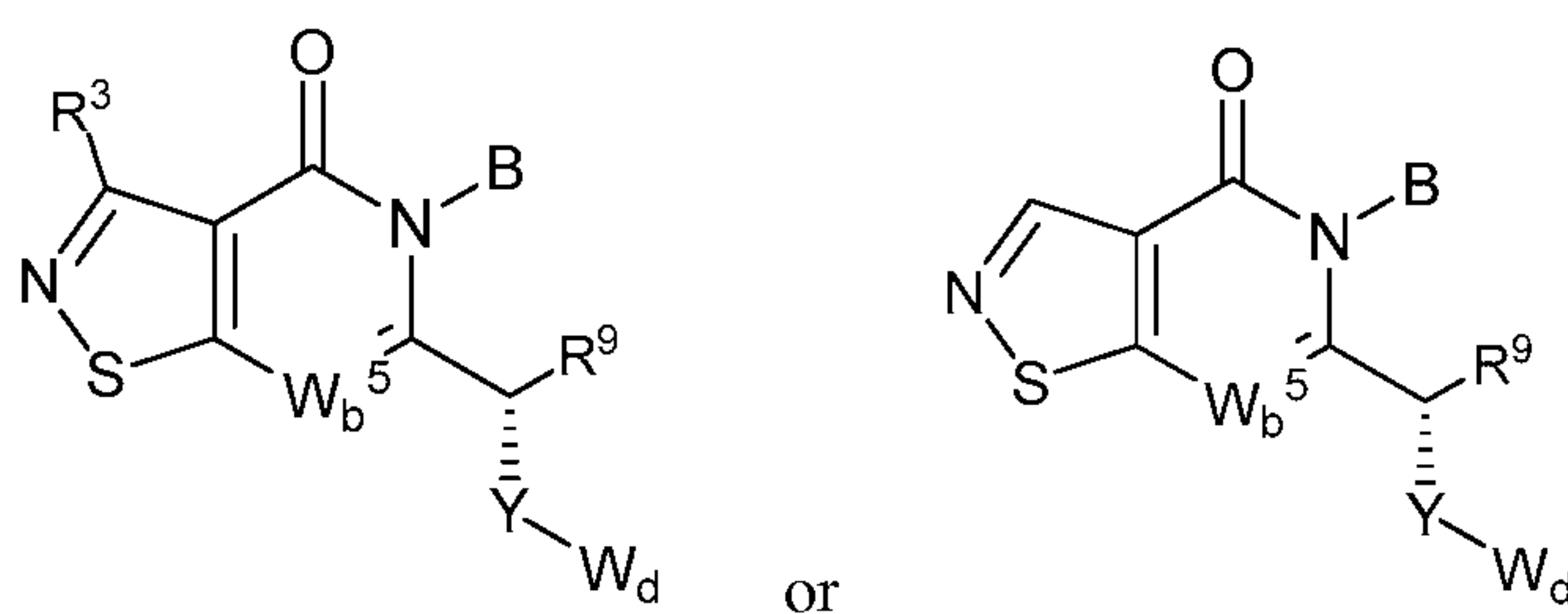
Formula (Va)
