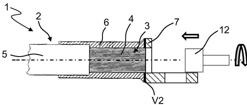
Fig. 2C
