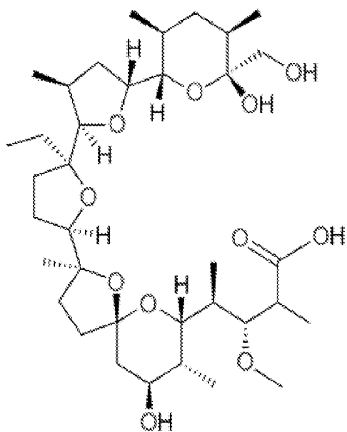
Monensin A
