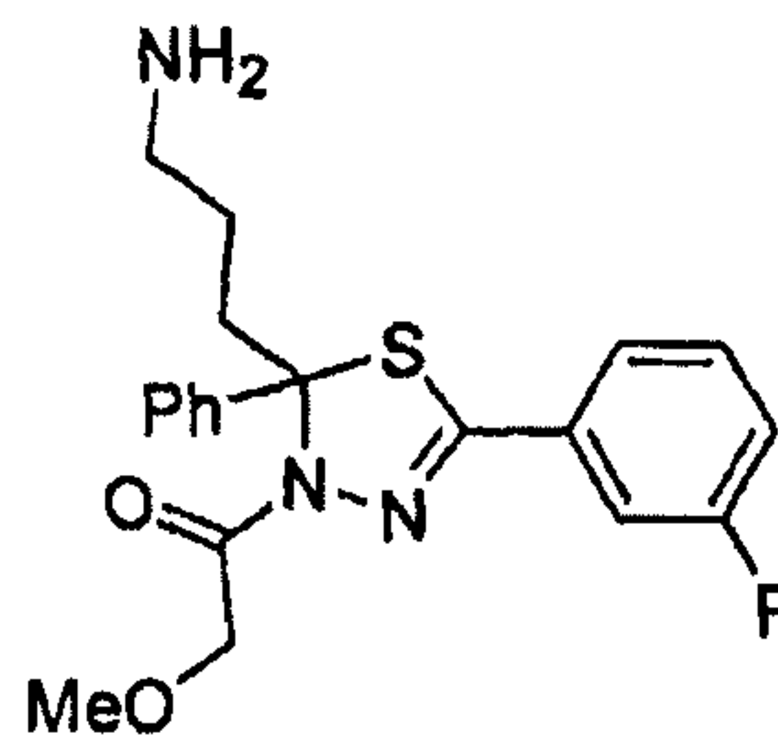
1-[2-(3-Aminopropyl)-5-(3-fluorophenyl)-2-phenyl-[1,3,4]thiadiazol-3-yl]-2- methoxyethanone
