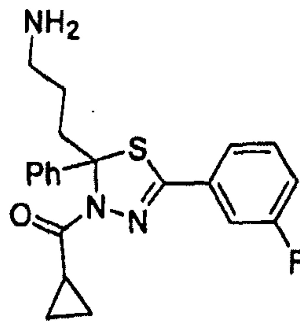
[2-(3-Aminopropyl)-5-(3-fluorophenyl)-2-phenyl-[1,3,4]thiadiazol-3-yl]- cyclopropylmethanone
