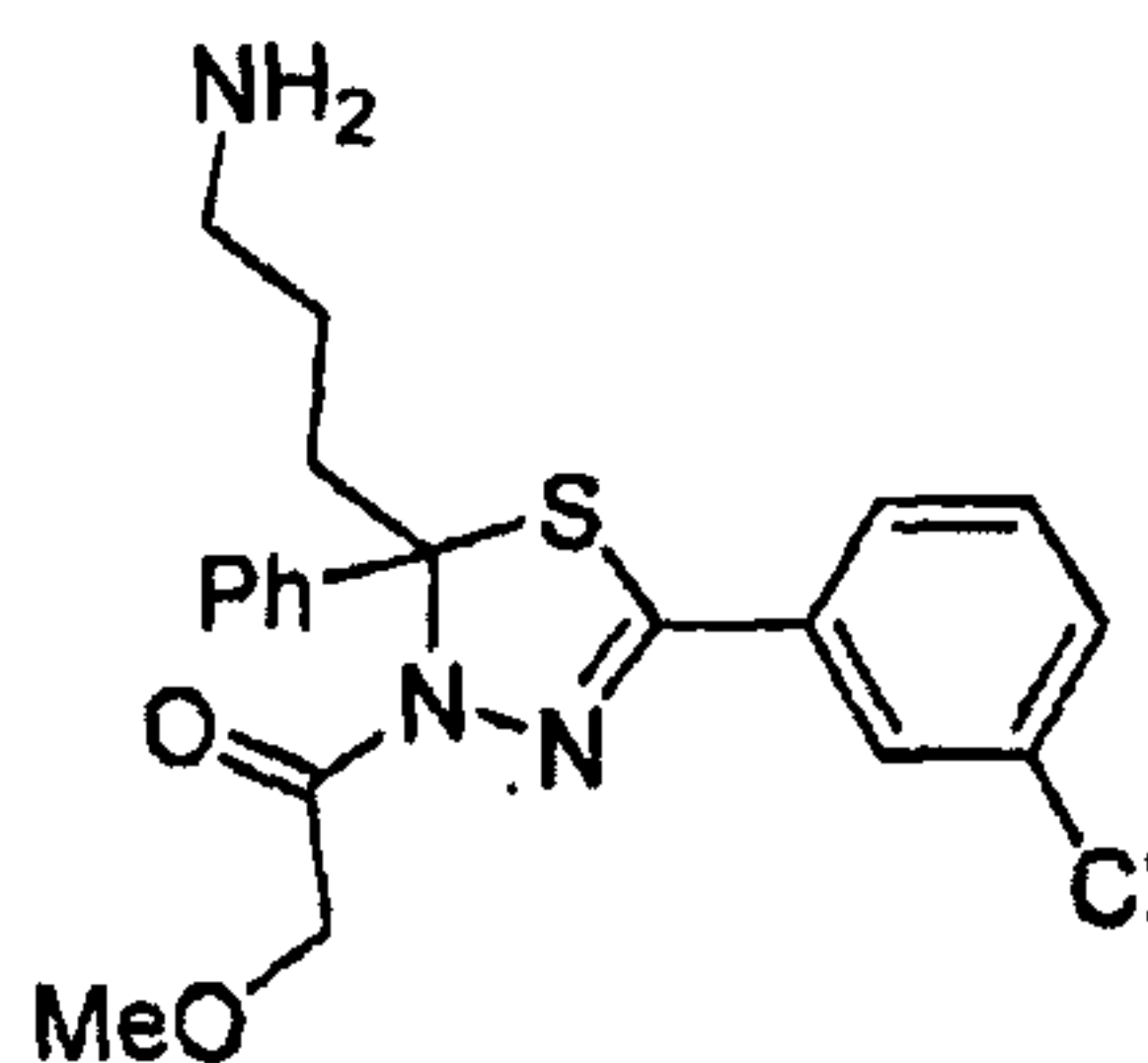
1-(2-(3-Aminopropyl)-5-(3-chlorophenyl)-2-phenyl-1,3,4-thiadiazol-3(2H)-yl)-2- methoxyethanone
