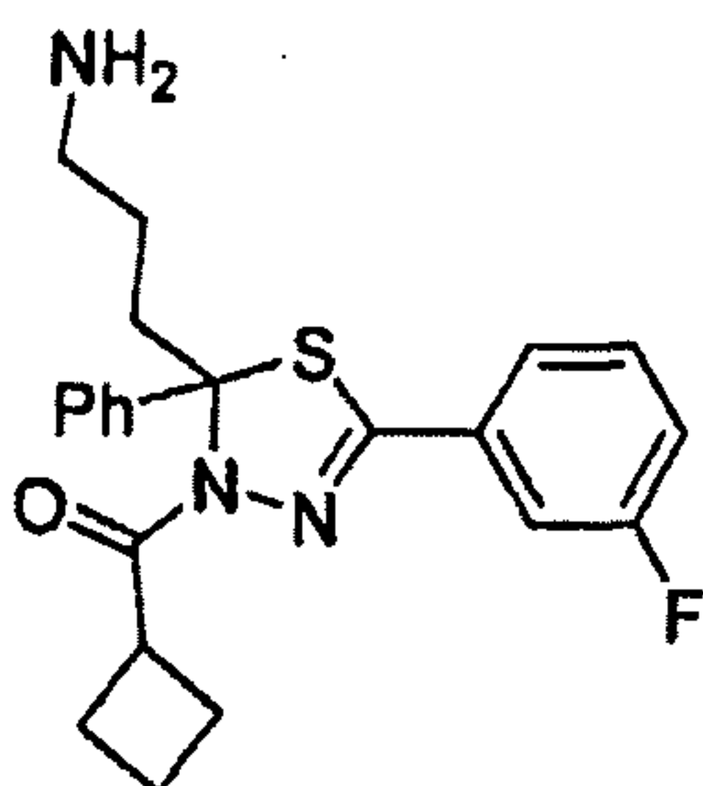
(2-(3-Aminopropyl)-5-(3-fluorophenyl)-2-phenyl-1,3,4-thiadiazol-3(2H)-yl)(cyclobutyl)methanone
