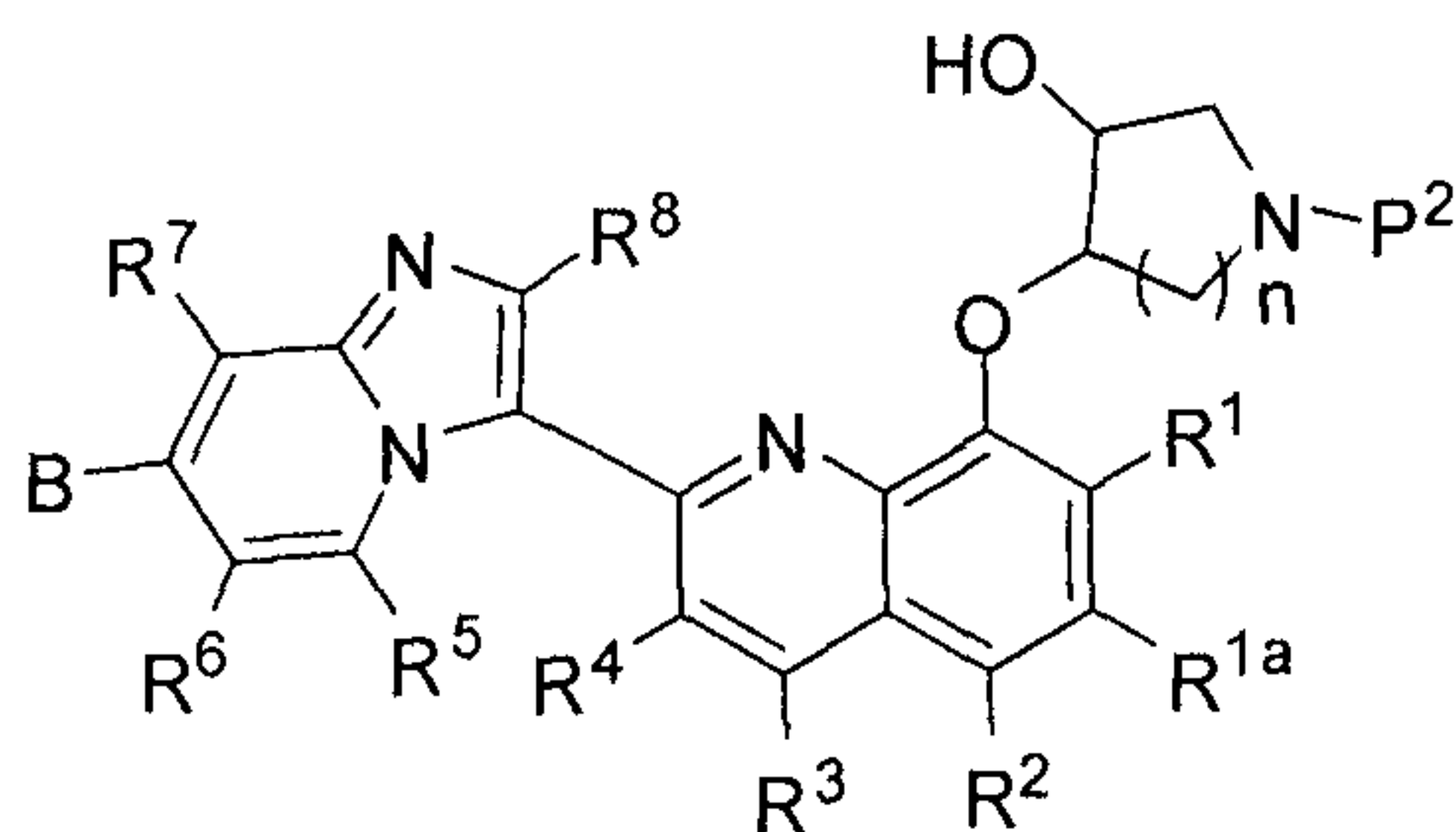
VII
