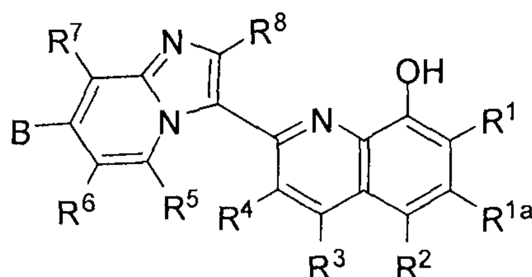
IV
