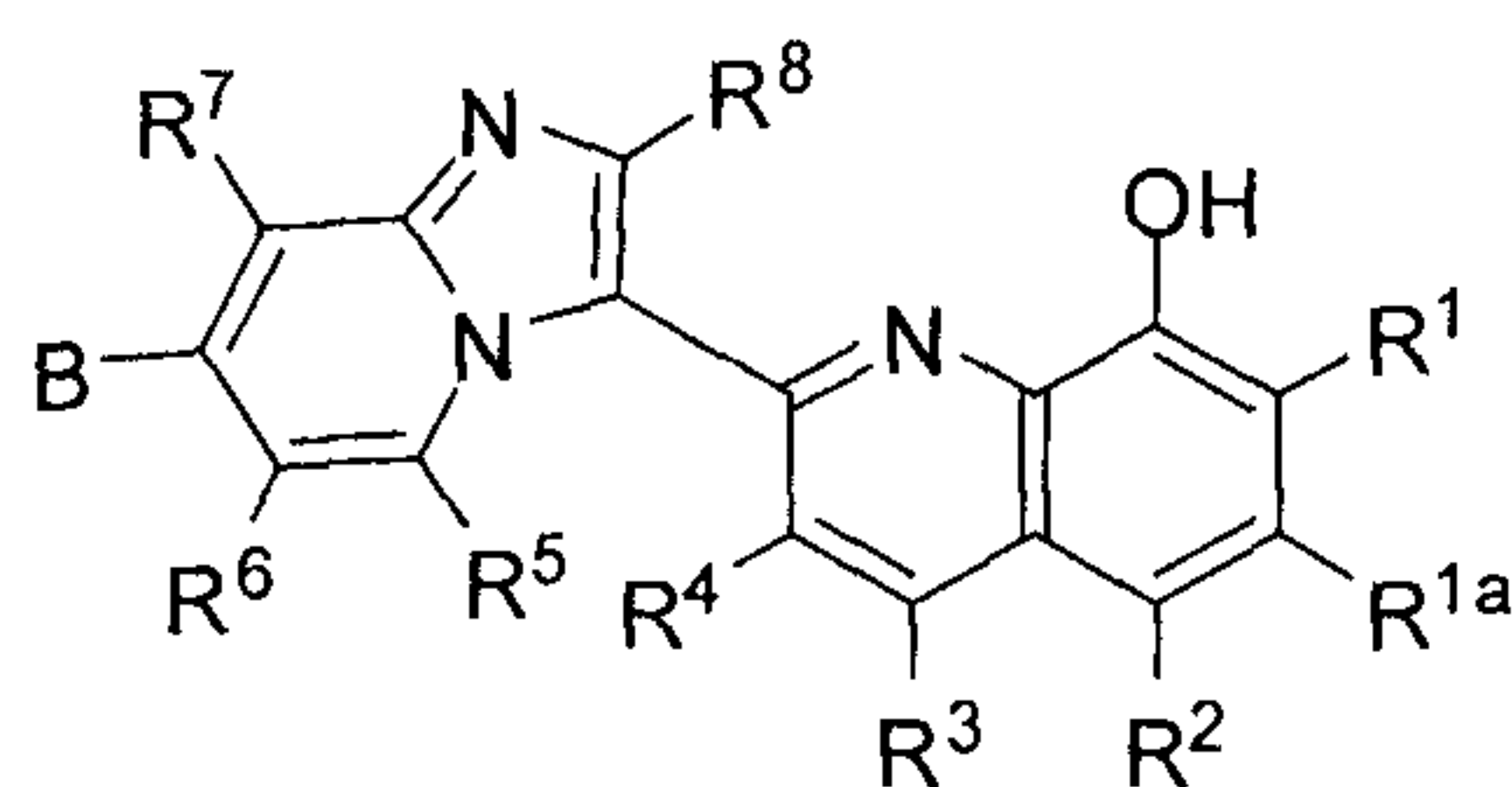
IV
