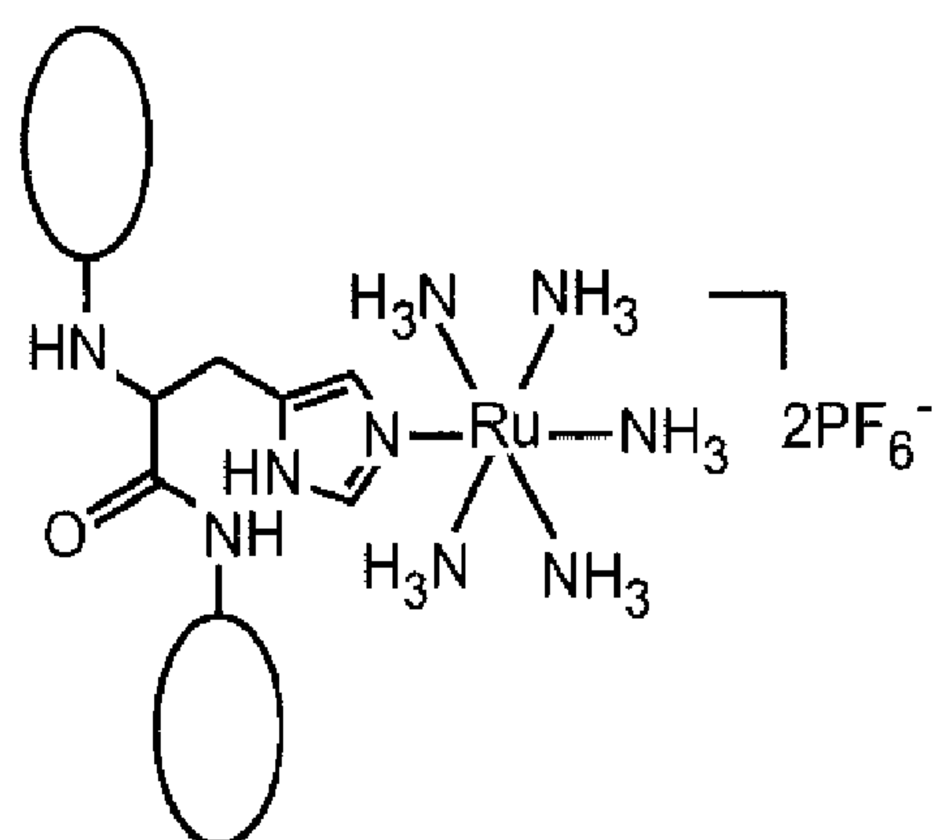
Pentaammine
