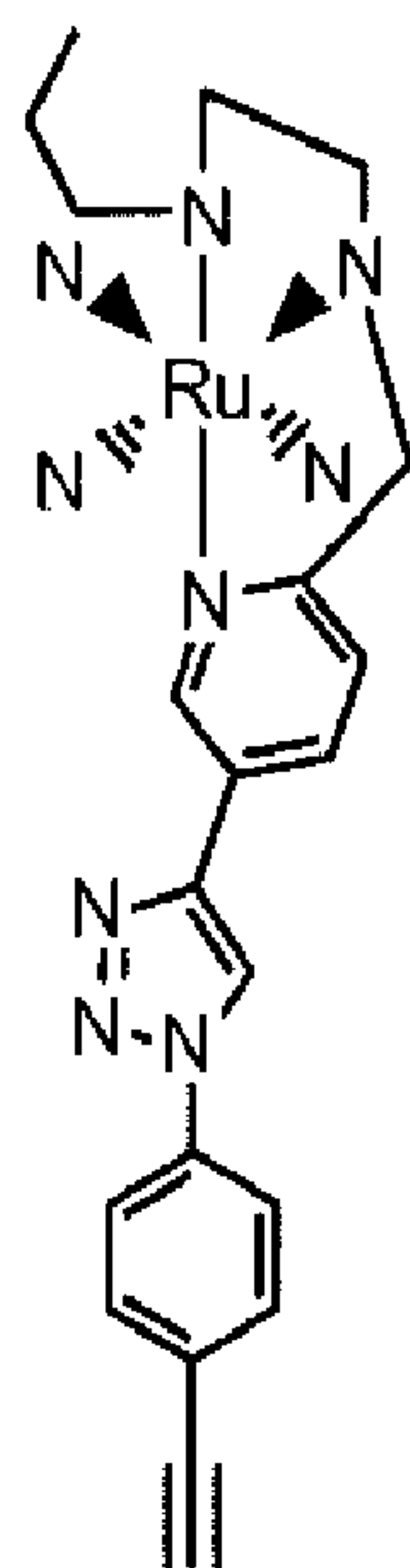
Tridentate
