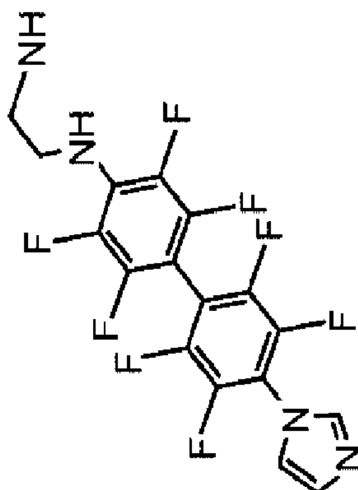
b. Amine
