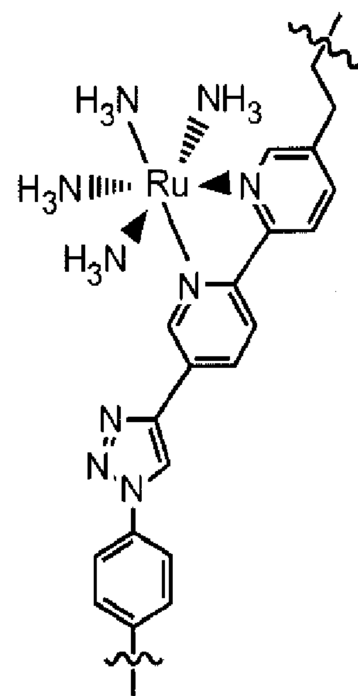
Bidentate
