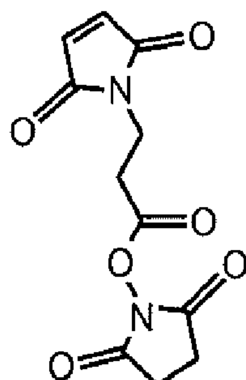
C3-Mal-NHS
