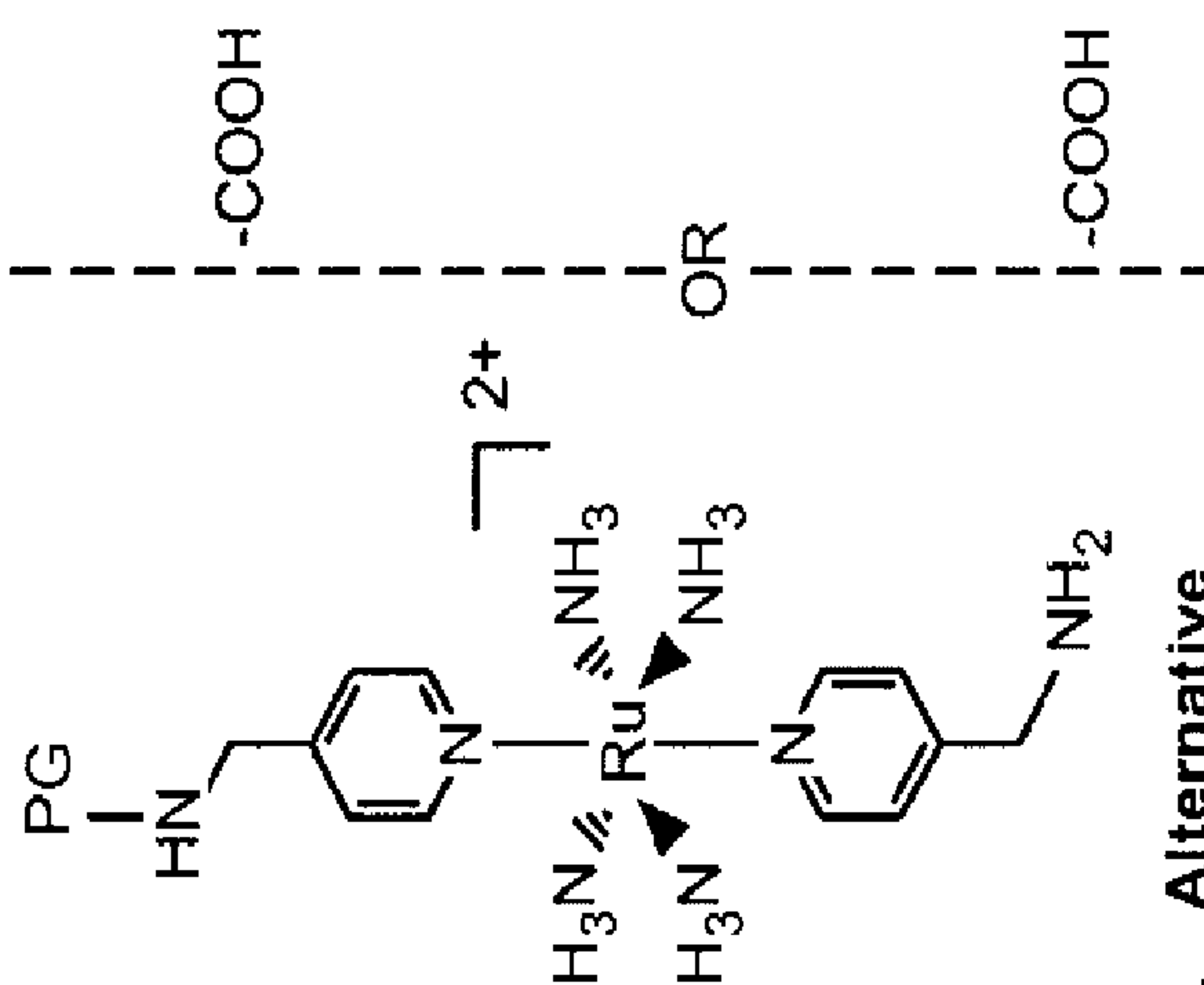
b. Amine
