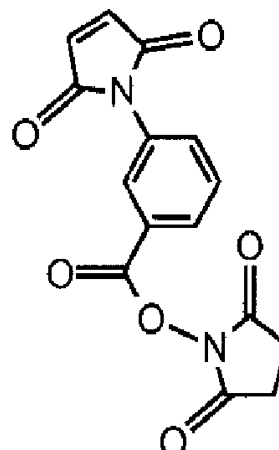
MBA-Mal-NHS
