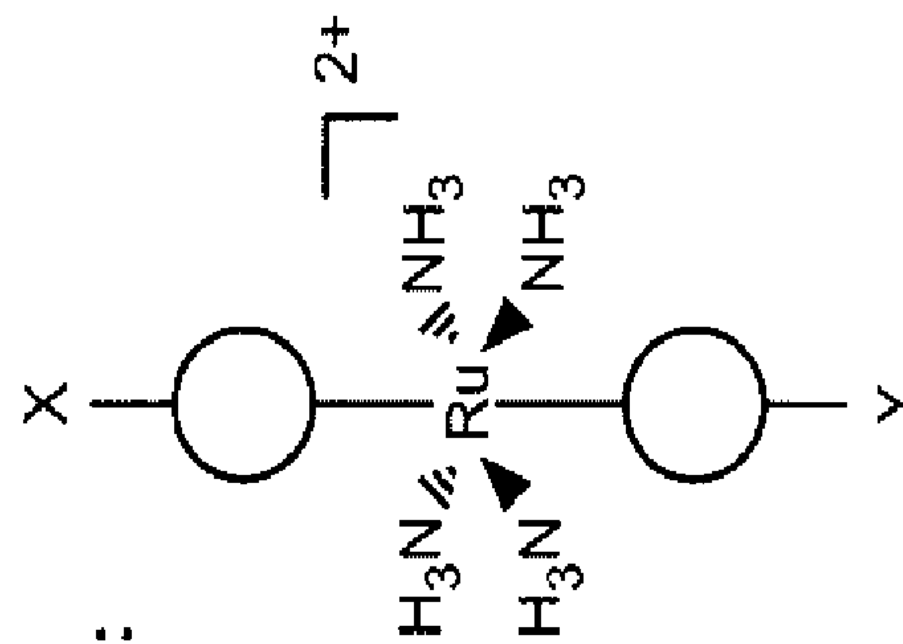
a. Coordination
