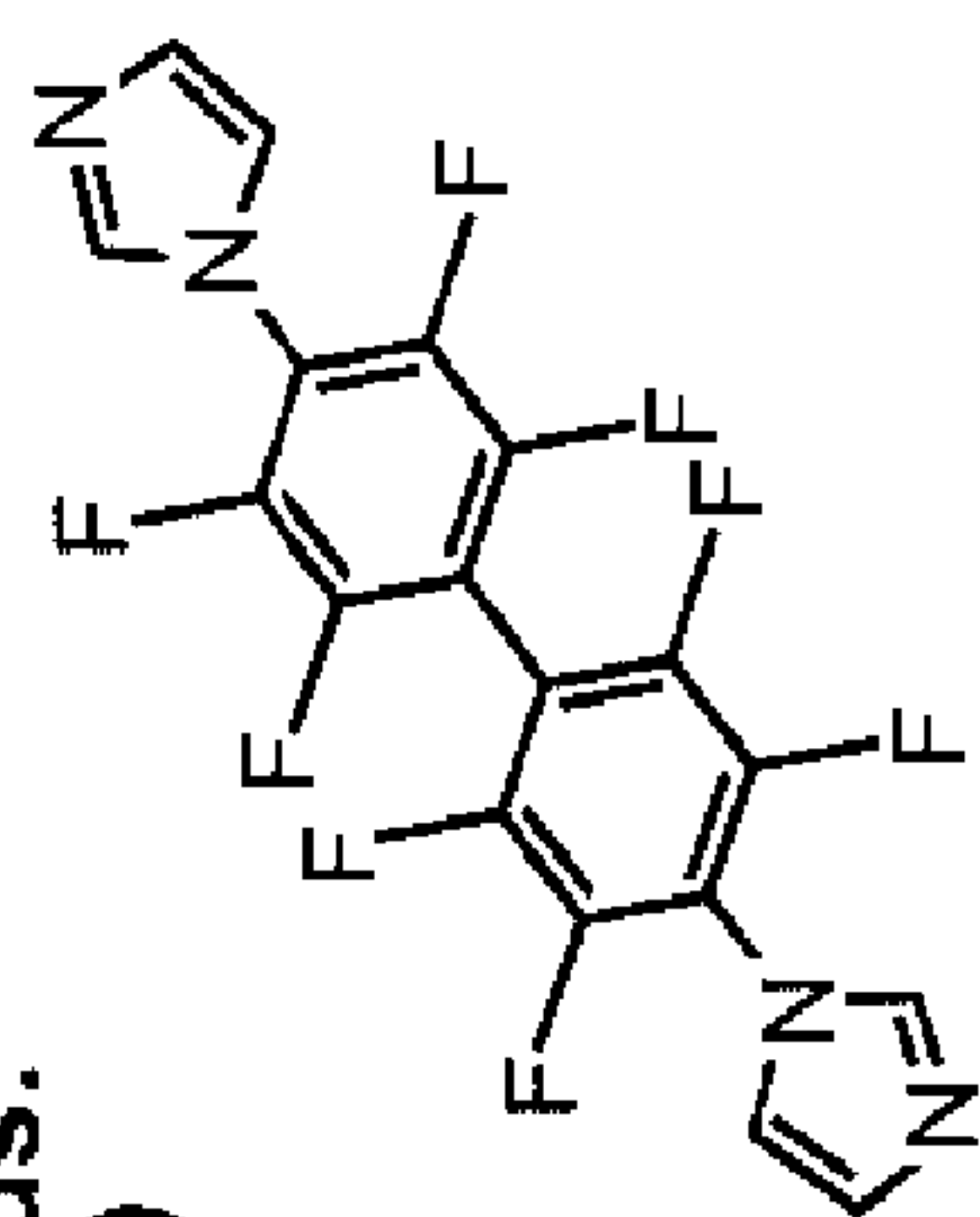
a. Coordination
