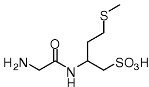
(I-Z): 2-(2-aminoacetamido)-4-(methylthio)butane-1-sulfonic acid;
