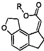
(Z)-X
