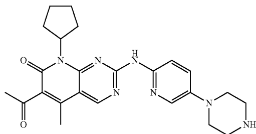
Palbociclib
