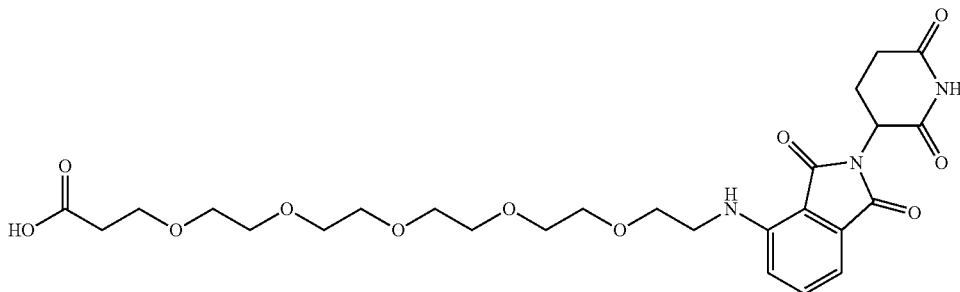
Linker 20: 3-(2-(2-(2-(2-(2,6-Dioxopiperidin-3-yl)-1,3-dioxoisindolin-4-yl)amino)ethoxy)ethoxy)ethoxy)propanoic acid
