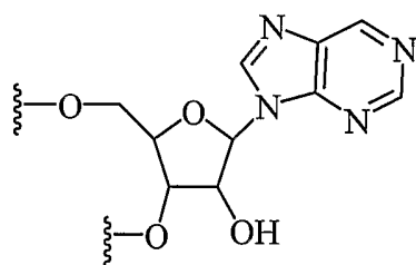
Purine (Pu)
