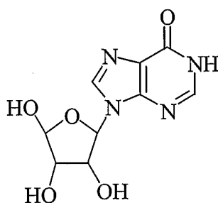
Inosine
