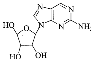
2-AminoPurine
