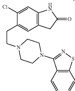
Ziprasidone
