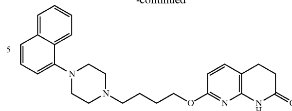
PF-00217830
