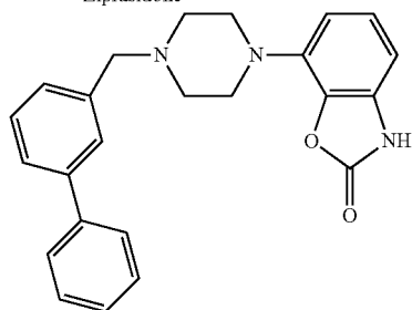
Bifeprunox
