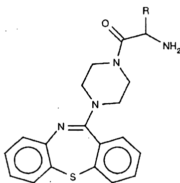
(XI)
