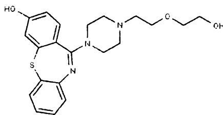
(7-OH-QTP),
