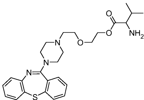
valine-quetiapine (Val-QTP)
