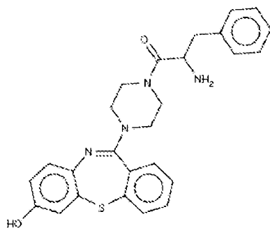
(VII),
