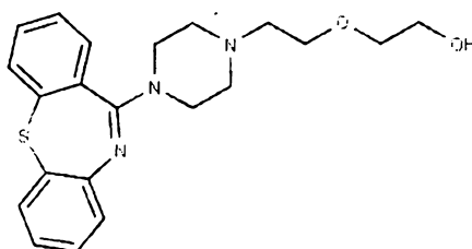
(QTP)
