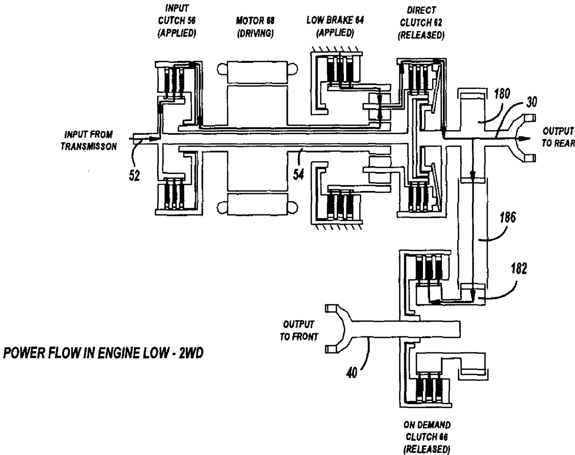
FIG. - 11C
