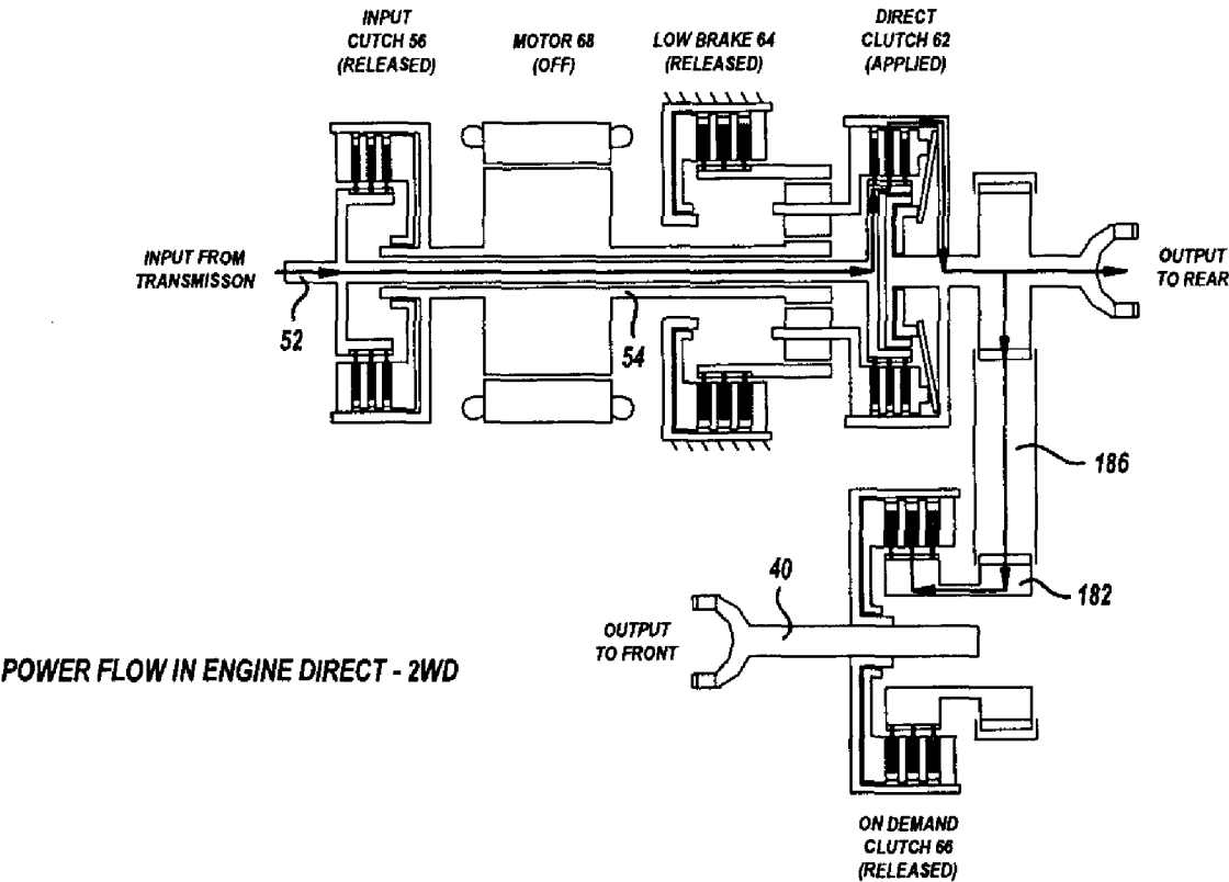
FIG. - 11E
