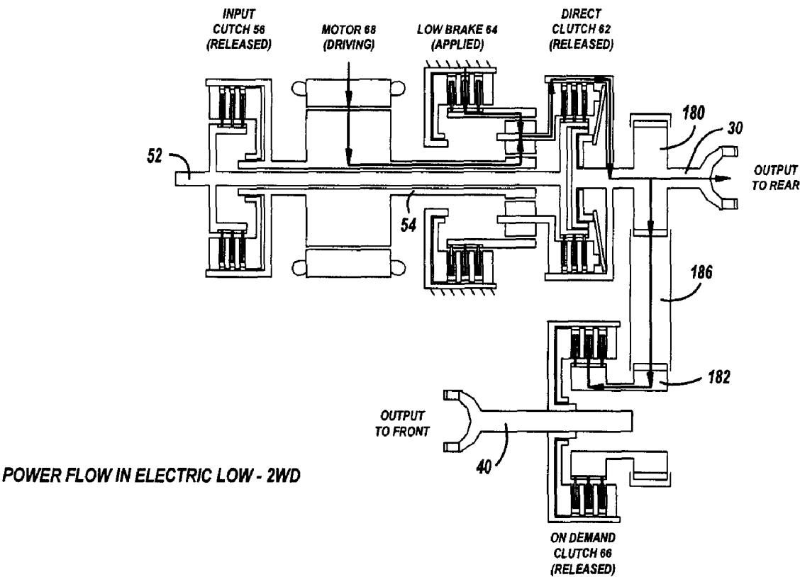
FIG. - 11A
