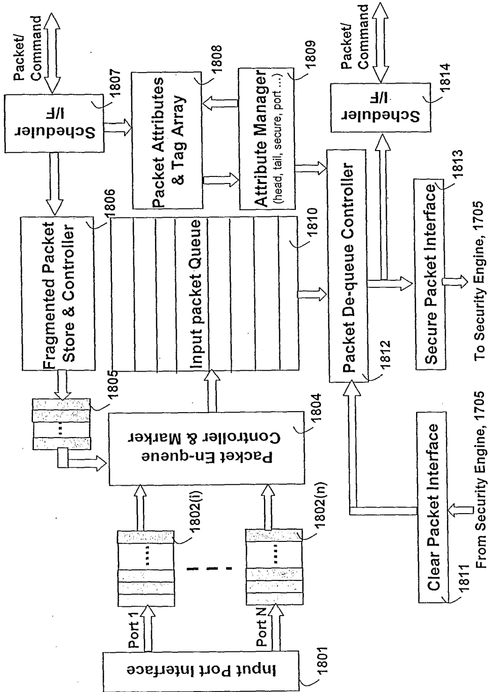
Fig. 18 Input Queue & Controller
