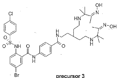
precursor 3
