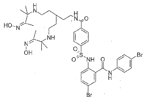
precursor 2
