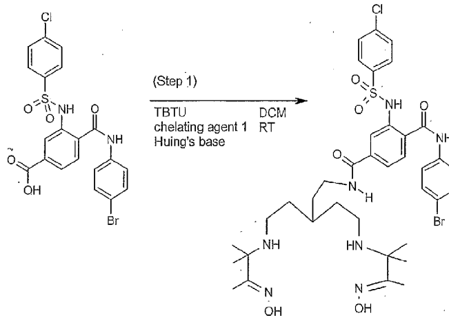
precursor 1
