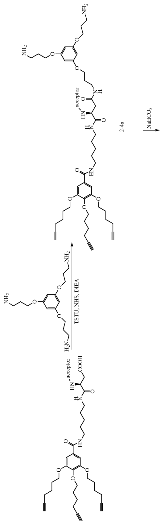
Schéme 19
