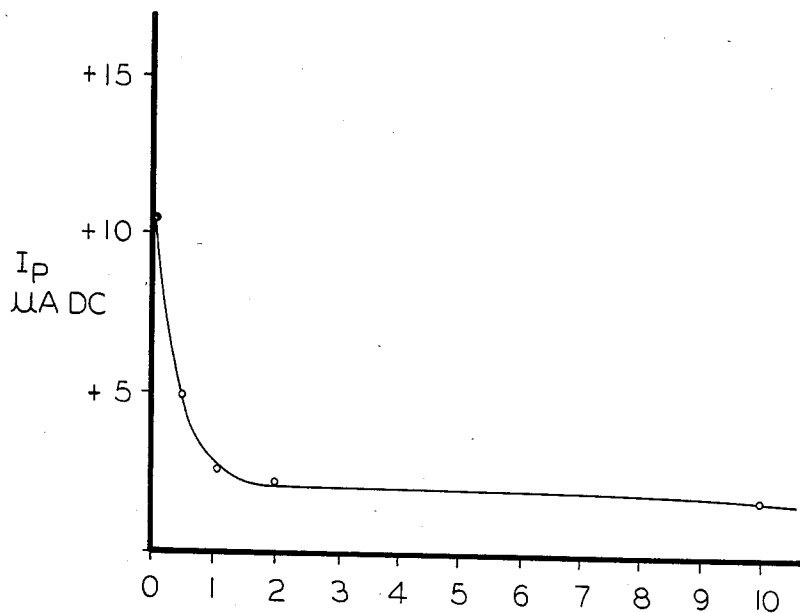
FIG. 3 R_S MEGOHMS
