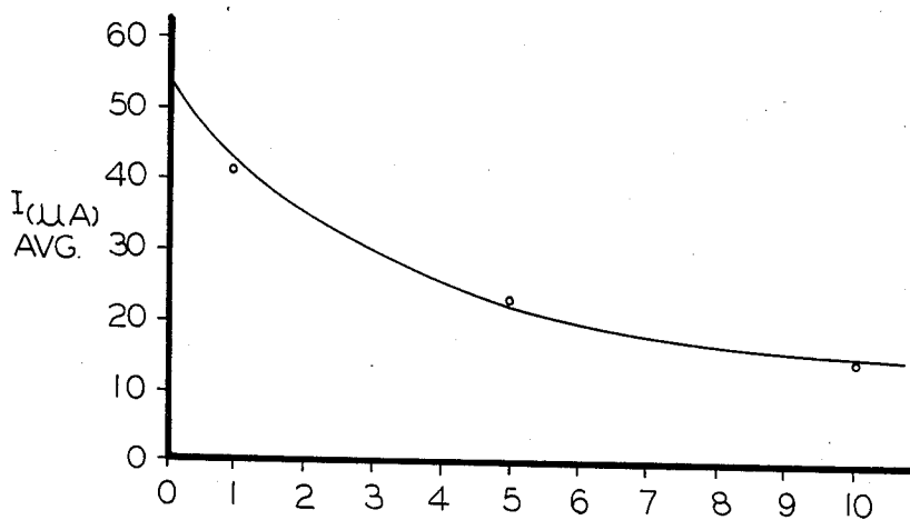
FIG. 4 R_S (MEGOHMS)
