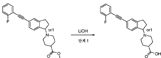
키랄 분리 2
