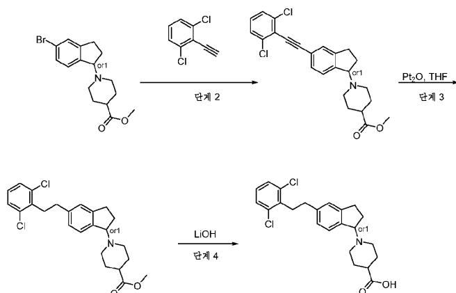
키랄 분리 1
