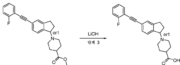
키랄 분리 1
