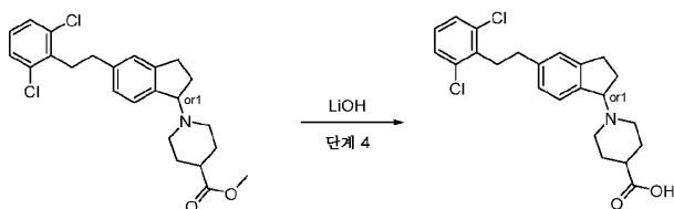
키랄 분리 2
