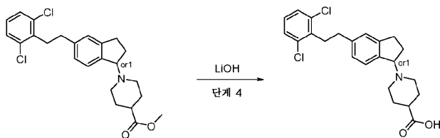
키랄 분리 1
