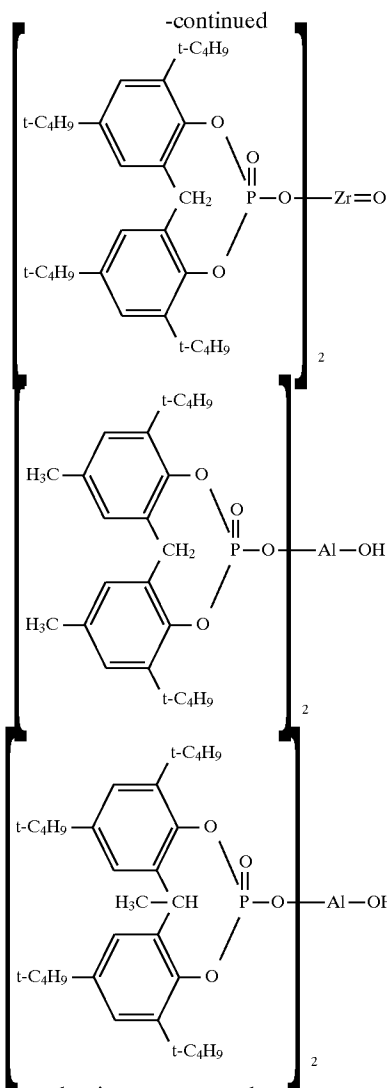
(d) Lithium aluminum compound
