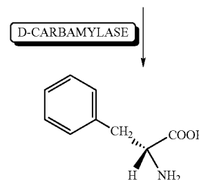
D-AMINO ACID
