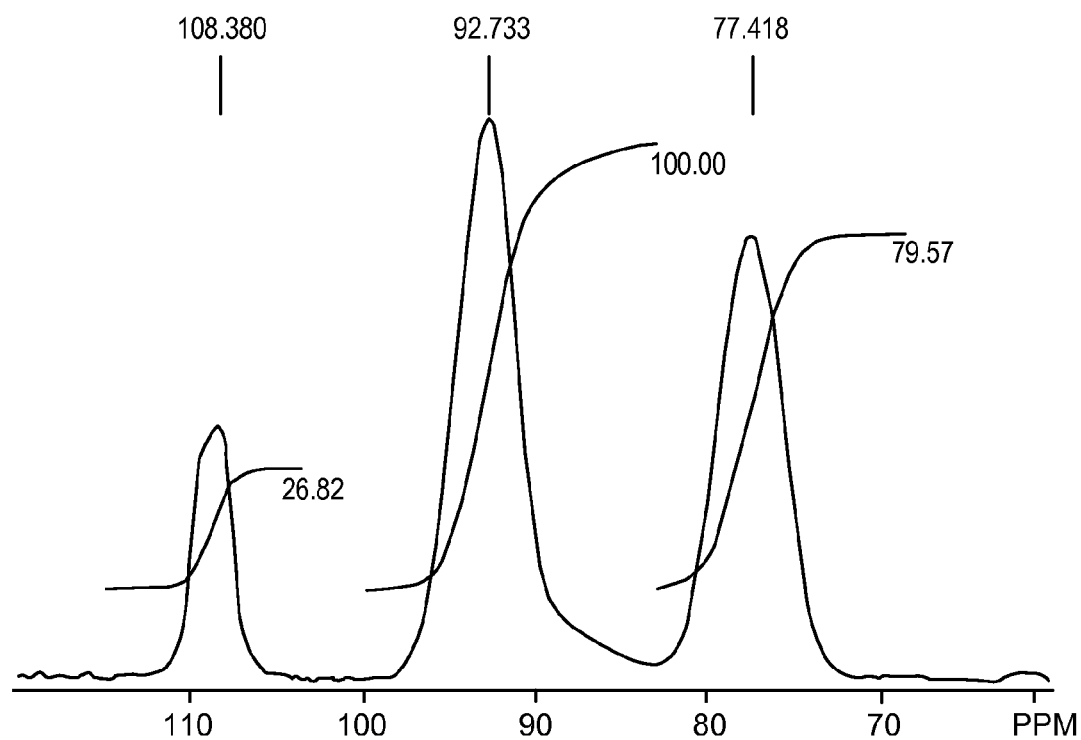
FIGURE 23A: LTPS ^{31}\text{P} NMR
