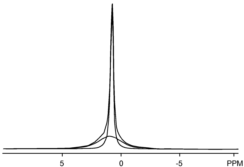
FIGURE 22A: LTPS ^7\text{Li} NMR
