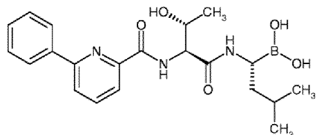
Delanzomib
