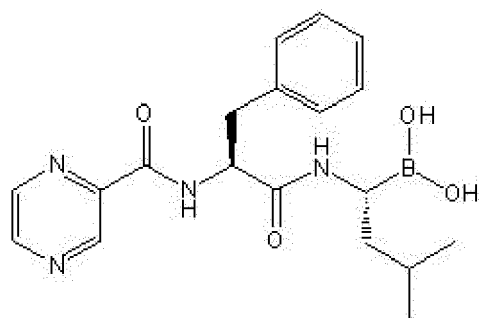
Bortezomib
