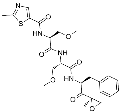
Oprozomib
