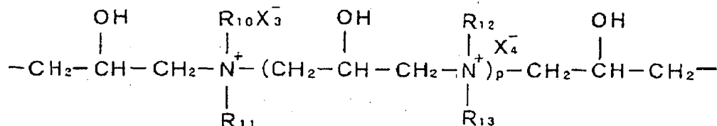
Formule générale (4)
