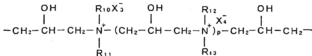
Allgemeine Formel (4)
