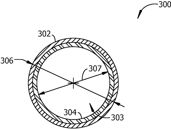
SECTION G - G Fig. 33
