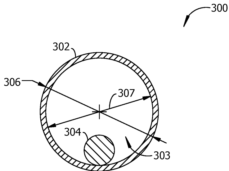
SECTION D - D Fig. 8
